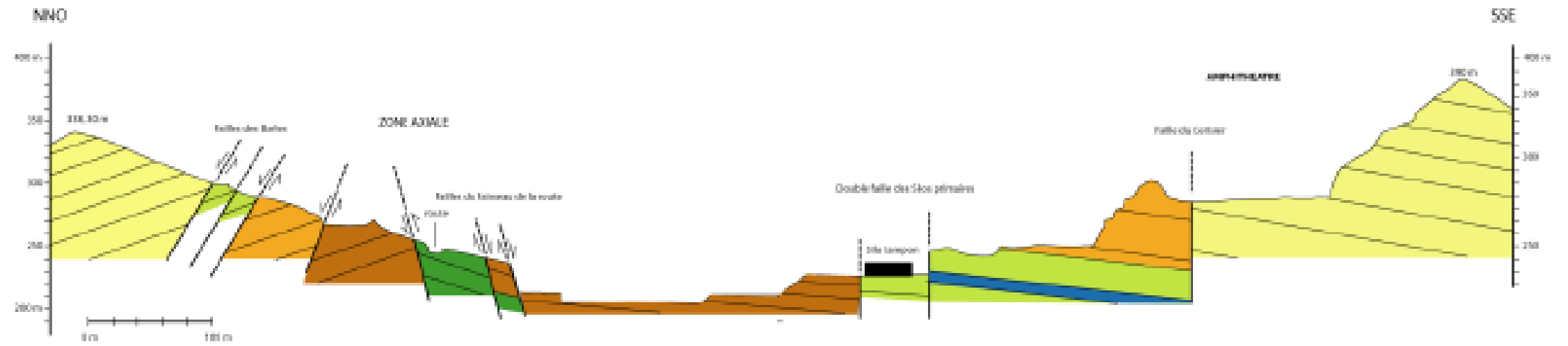
Figure 17. Profils géologiques transversaux montrant la structure du dôme et ses accidents.
